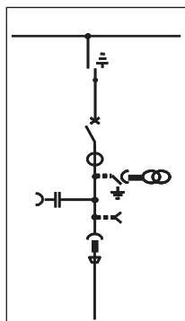
断路器柜
