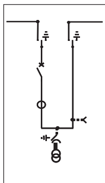
母线联络开关柜
