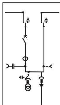
母线联络开关 带出线柜
